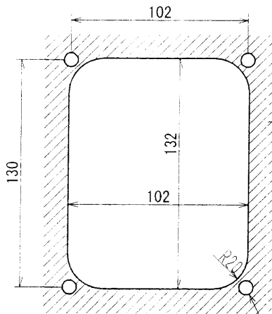
取付穴寸法 CUTOUT DIMENSIONS
