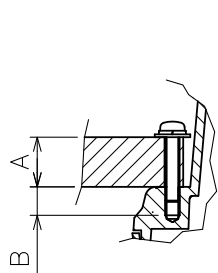
取付ネジ部断面 尺度 1/2 DETAIL FOR FASTENING (SCALE: 1/2)
